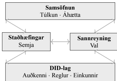
Figure 1: Fjöгурra laga byggingarlist RSN.
