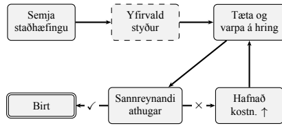
Figure 3: Líftími staðhæfingar með ítrunarlykkju.
